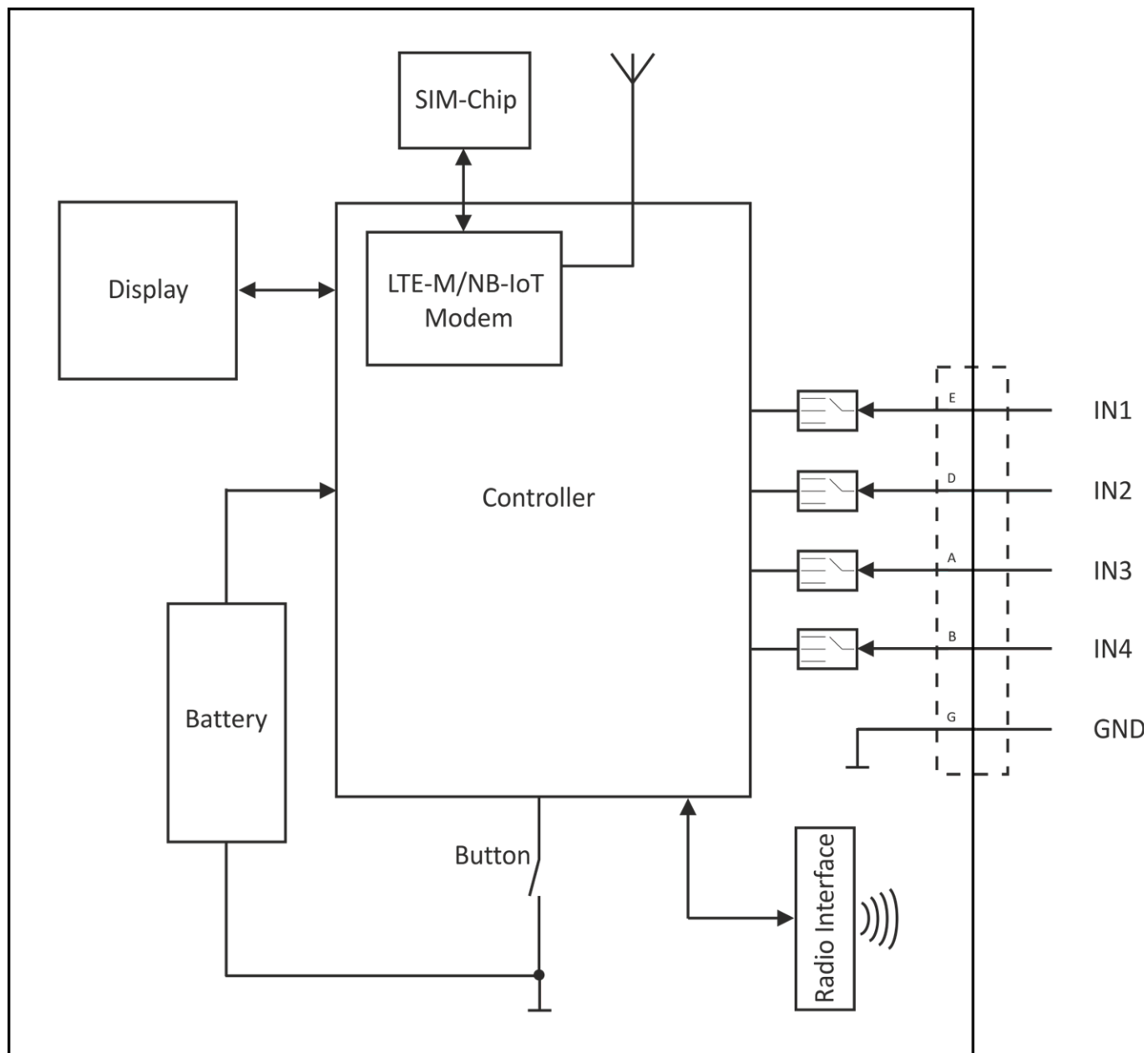
Blockschaltbild des D022-4Z0012xxx05 (Type Key D022-4Z00121L905)
