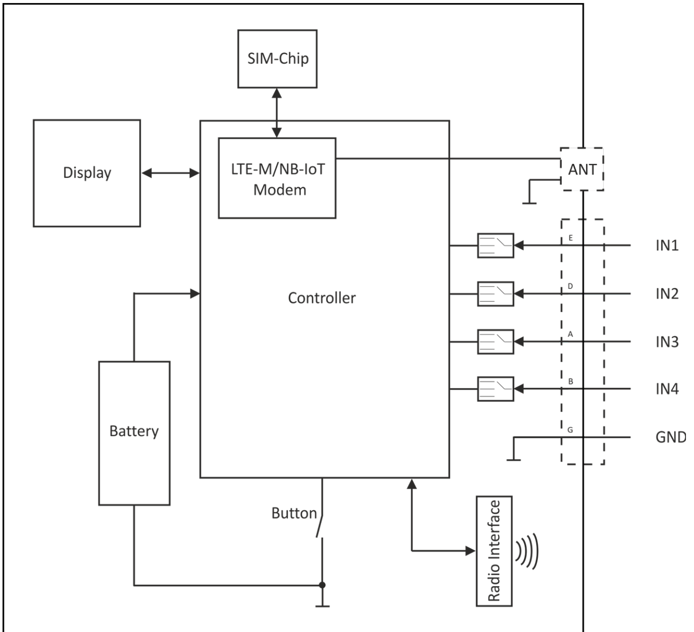
Blockschaltbild des D022-4Z0012xxx05 (Type Key D022-4Z0012 00D 05)
