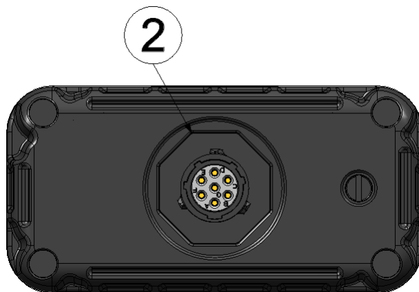
Unterseite des D022-4Z0012xxx05 (Type Key D022-4Z00121L905)
