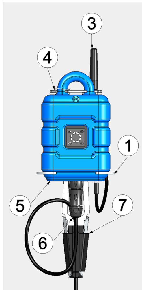
Wandmontage Schritt 2
