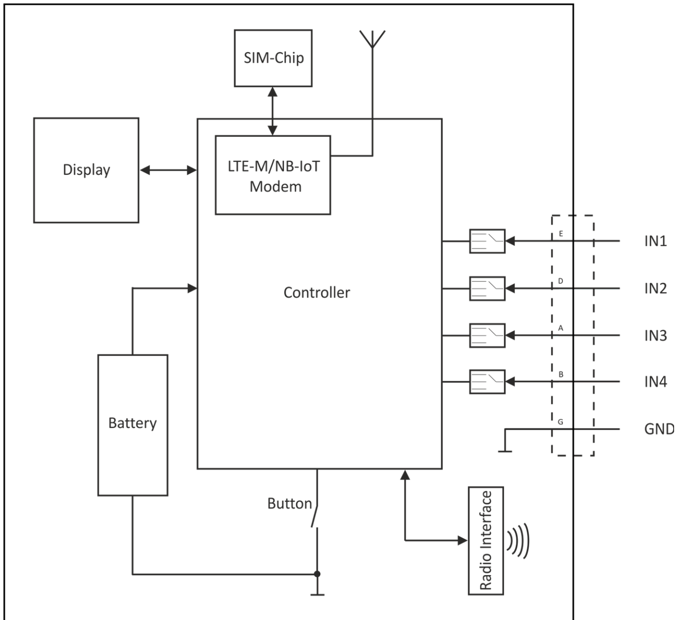
Blockschaltbild des D022-3Z0012xxx05 (Type Key D022-3Z00121L905)
