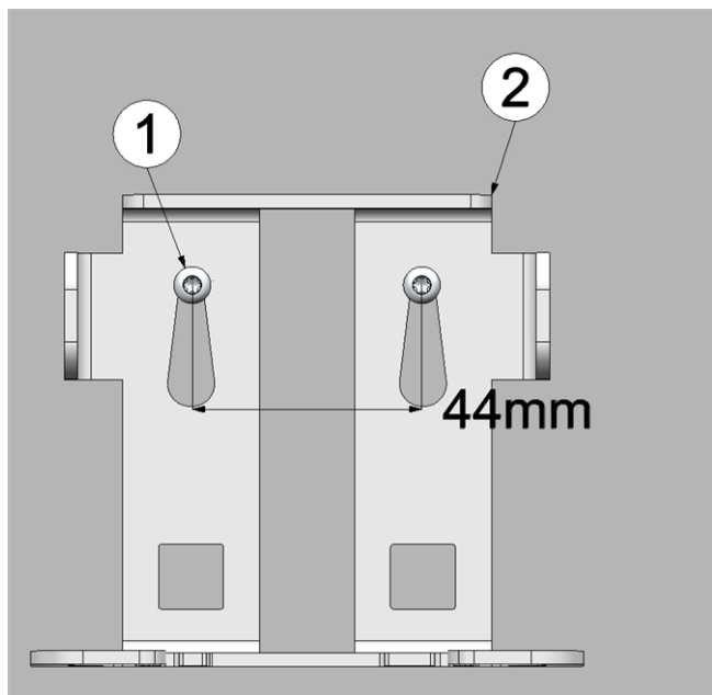
Wandmontage Schritt 1
